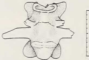
Abb. 2: Schwanzwirbel von Gallotia goliath (G1) mit je zwei transversalen Fortsätzen, die eines der Gattungsmerkmale für Gallotia sind. Maßstab: 10 mm.
